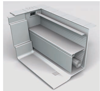
Rollladenschacht Inline
