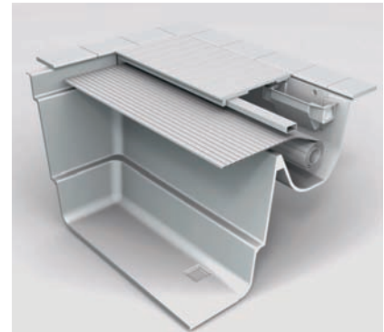
Rollladenschacht Classic
