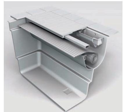
Rollladenschacht Integra
